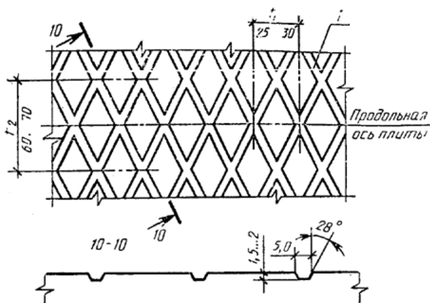
1 - рифление рабочей поверхности плиты
